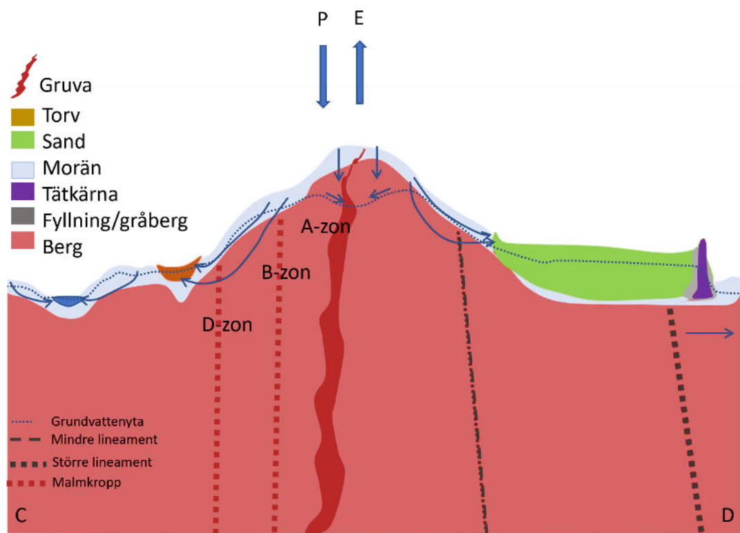
Figur 5-7. Typprofil över det lokala området utmed profil C-D från Viscariaområdet sydvästra till nordöstra del. Typprofilens sträckning i plan visas i Figur 5-5.
