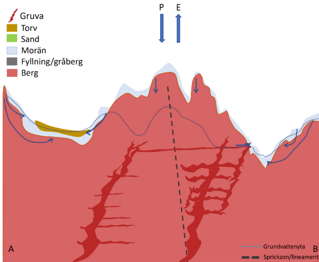
Figur 5-6. Typprofil över det lokala området utmed profil A-B, från området nordväst om Viscaria till sydöst. Typprofilens sträckning i plan visas i Figur 5-5.
