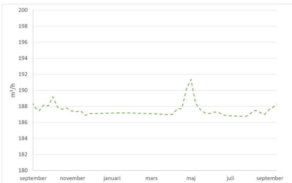
Figur 10-22. Beräknat inflöde till gruvan vid tömning av gruvan i AB-zonen simulerat för ett normalår. Då gruvan var i drift observerades ett inflöde på 150–200 m 3 /h, medelvärdet för det beräknat inflödet för ett hydrologiskt år 187 m 3 /h.
