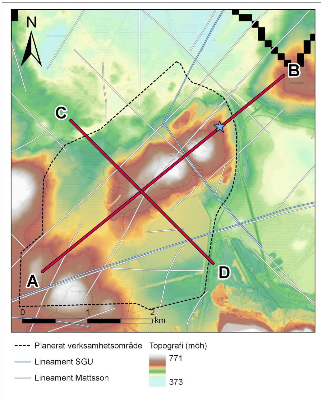
Figur 5-5. Läge för de typprofil över topografi, jordarter och områdets större sprickzoner som visas i Figur 5-6 (typprofil A-B) och Figur 5-7 (typprofil C-D). Den blå stjärnan markerar området där grundvatten från den vattenfyllda gruvan strömmar ut.
