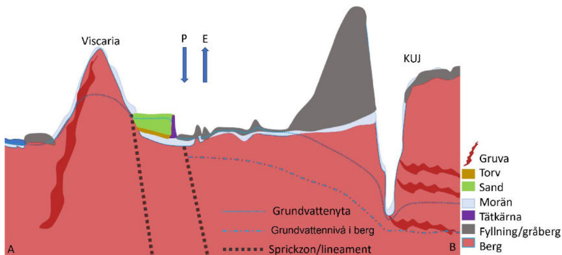
Figur 5-4. Typprofil över det regionala området från nordväst om Pahtajoki, över Peuravaara där Viscariagruvan ligger och vidare mot området kring Kirunavaaragruvan (KUJ) där gråbergssupplaget syns som en tydlig höjd och dagbrottet syns som en tydlig sänka i profilens högra del. Typprofilens sträckning i plan visas i Figur 5-3 (A-B).
