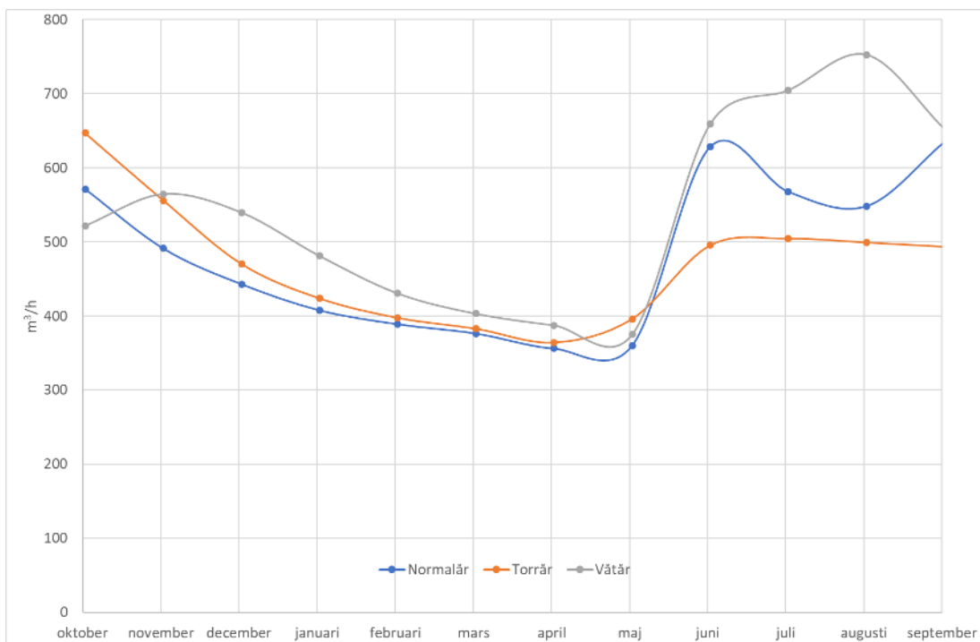
Figur 11-35. Totalt inflöde till underjordsgruva och dagbrott i för normalår, torrår och våtår.
