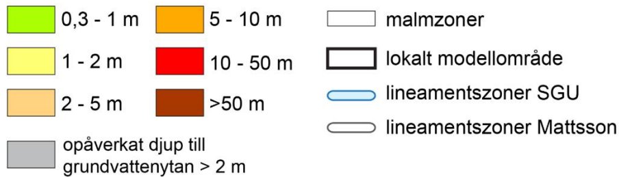
Figur 11-23. Påverkansområde vid tömning av befintlig gruva och vid fullt utbruten gruva i Fas 3, torrår. Påverkade områden med större djup till grundvattenytan än 2 m under opåverkade förhållanden är gråmarkerade.
