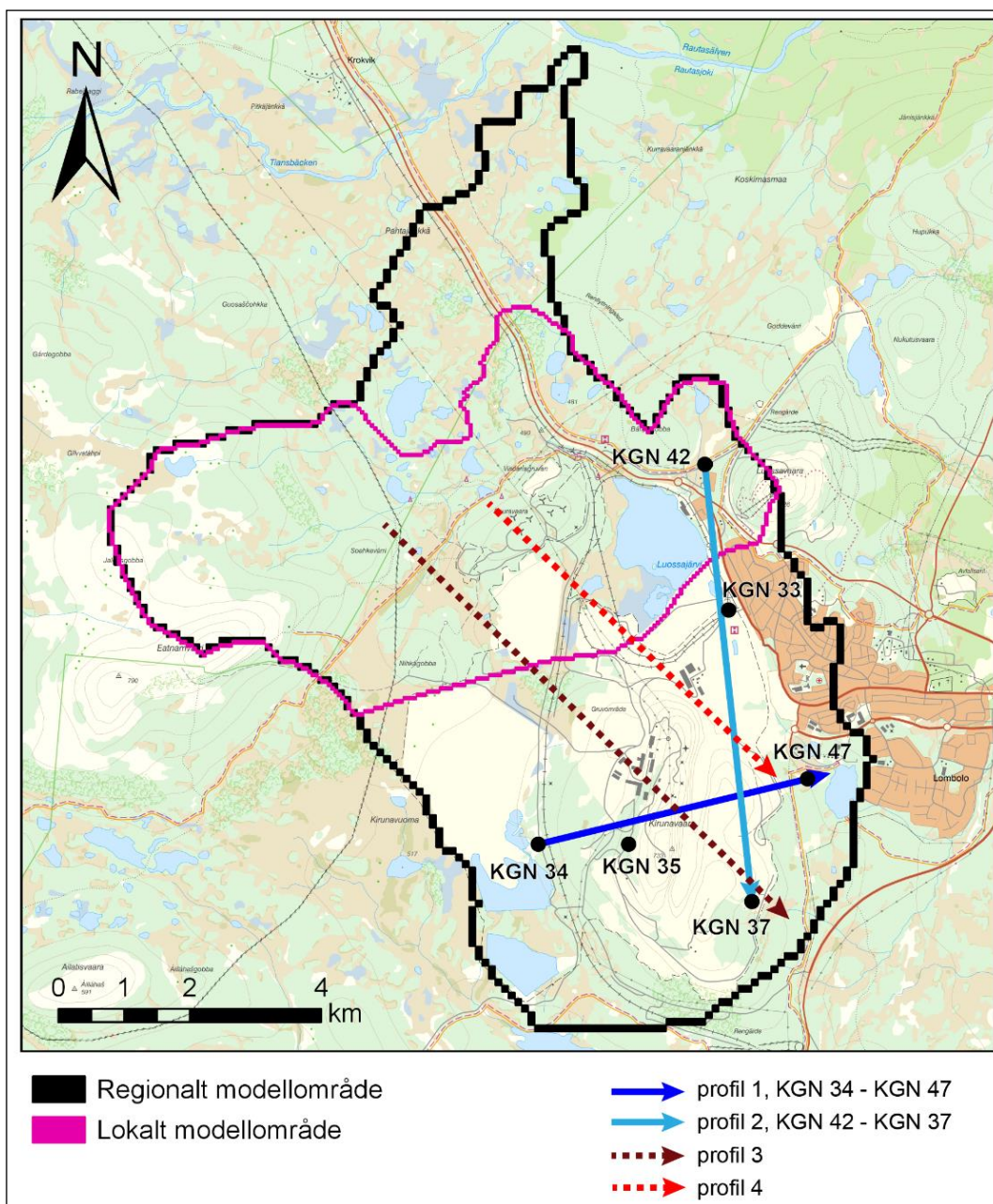
Figur 10-1. Profiler för vilket det redovisas beräknade resultat för grundvattennivå på olika djup i berget och för fria grundvattentytans läge i Figur 10-2 till och med Figur 10-7.
