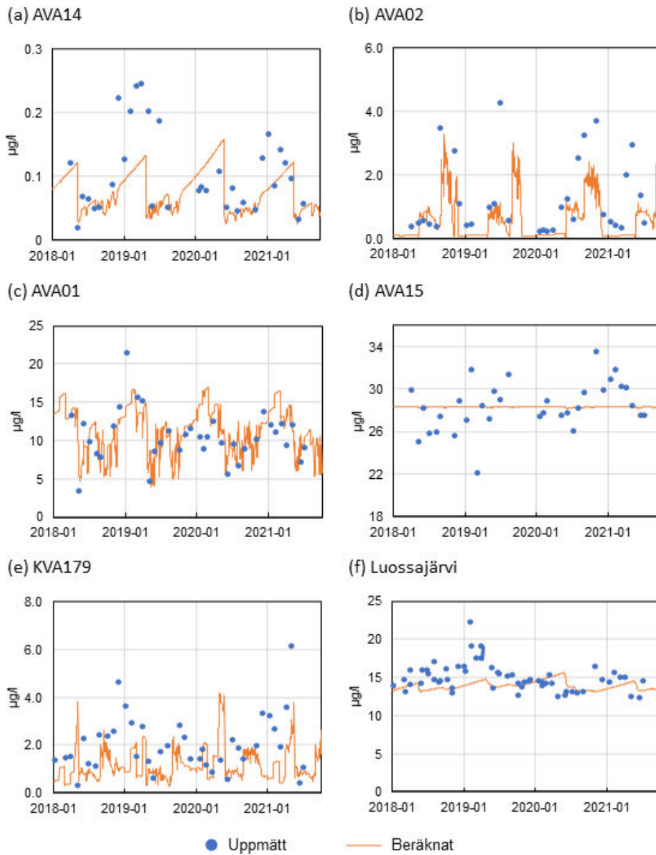
Figur 8-10. Uppmätta och beräknade halter uran (U) ( \mu\text{g/l} ): (a) AVA14, (b) AVA02, (c) AVA01, (d) AVA15, (e) KVA179 och (f) Luossajärvi.
