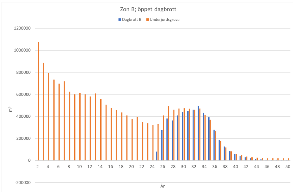
Figur 11-41. Inflödande vattenvolymer ( m^3/\text{år} ) till dagbrott och underjordsgruva i B-zonen för fallet med öppna dagbrott. Om nettoflödet är positivt sker en inströmning av vatten, om det är negativt sker en utströmning av vatten.
