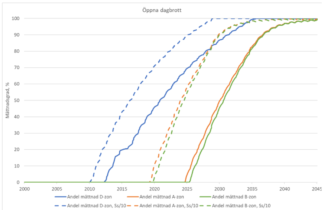
Figur 11-37. Återmättnadsförlopp i fallet med öppna dagbrott. Figuren visar andelen av dagbrotten som är vattenfyllda i förhållande till tröskelnivån, dvs den nivå där ytvatten börjar flöda ut ur dagbrottssjöarna. Ss/10 hänvisar till de beräkningsfall där magasinstelet dividerats med en faktor 10 i bakgrundsberg och sprickzoner.
