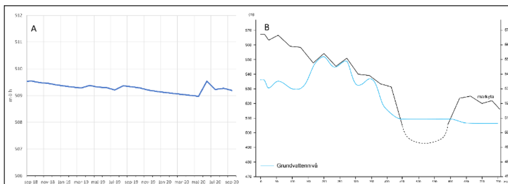
Figur 10-21. Tidsserie över den beräknade vattenytan i den kollapsade delen av gruvan (A) samt en profil som visar den beräknade fria grundvattentytans läge från ca 400m SV om gropen till 150 m NO om gropen (B).
