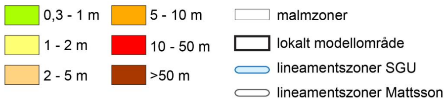
Figur 11-22. Påverkansområde vid tömning av befintlig gruva och vid fullt utbruten gruva i Fas 3, torrår.
