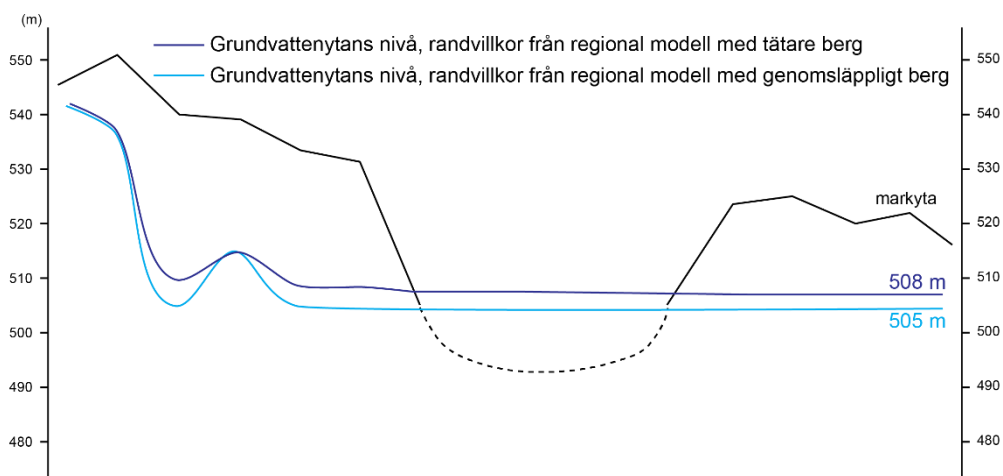
Figur 10-11. Grundvattentyta genom den kollapsade delen av gruvan för ett fall med tät berg som ledde till en felaktig påverkan från regionalmodellen och ett med tät berg och korrigerad påverkan från regionalmodellen.
