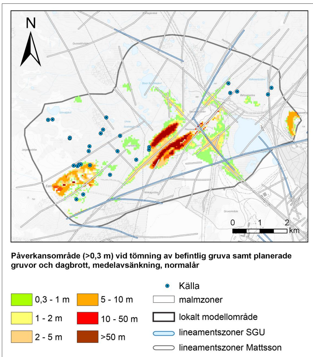
Figur 11-20. Påverkansområde vid tömning av befintlig gruva och vid fullt utbruten gruva i Fas 3, normalår. I figuren visas även fältkontrollerade källor i området.
