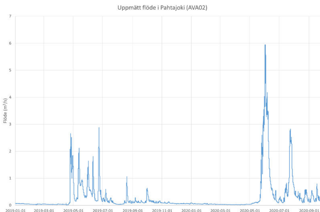
Figur 5-1. Flödestoppar i Pahtajokki under snösmältningen när tjälen fortfarande ligger kvar i marken.
