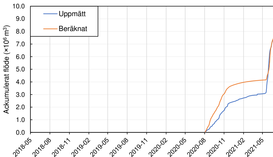
Figur 8-4. Uppmätta och beräknade flöden vid AVA14. (a) Hydrograf ( \text{m}^3/\text{s} ) (b) Ackumulerat flöde ( \times 10^6 \text{m}^3 ).
