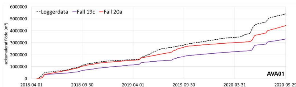
Figur 10-12. Jämförelse mellan ackumulerat flöde i AVA01 för fall 19c och fall 20a: före och efter adderingen av ett flöde från ledningen från Luossajärvi.
