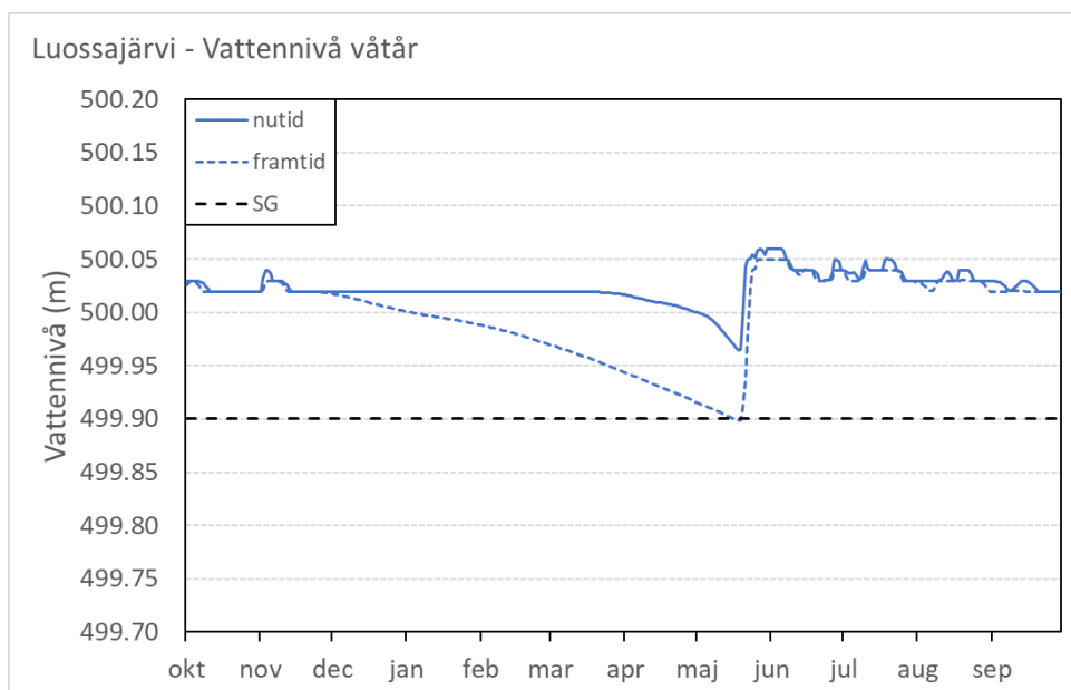
Figur 9-4. Jämförelse av förändringen i vattennivån i Luossajärvi för nutids- (heldragen blå linje) och framtidsscenarioer (streckad blå linje) för ett våtår i förhållande till sänkingsgränsen (SG – streckad svart linje).
