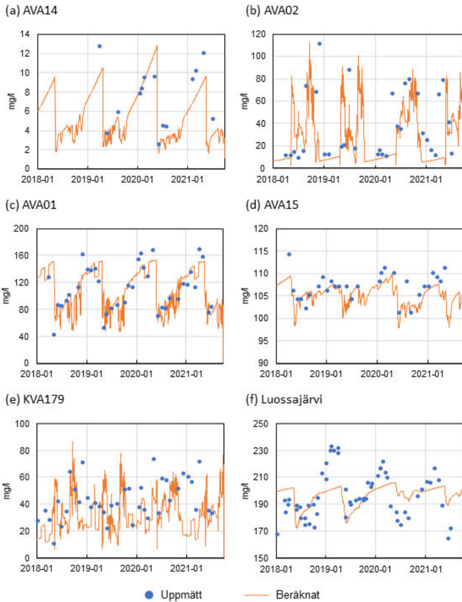
Figur 8-12. Uppmätta och beräknade halter av kalcium (Ca) (mg/l): (a) AVA14, (b) AVA02, (c) AVA01, (d) AVA15, (e) KVA179 och (f) Luossajärvi.
