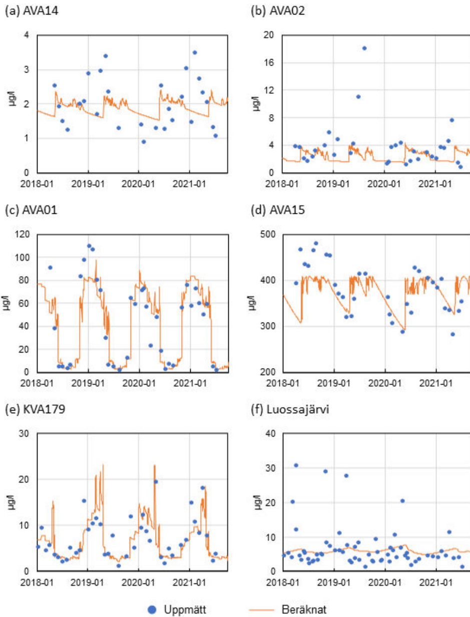
Figur 8-9. Uppmätta och beräknade zink (Zn) halter ( \mu\text{g/l} ): (a) AVA14, (b) AVA02, (c) AVA01, (d) AVA15, (e) KVA179 och (f) Luossajärvi.
