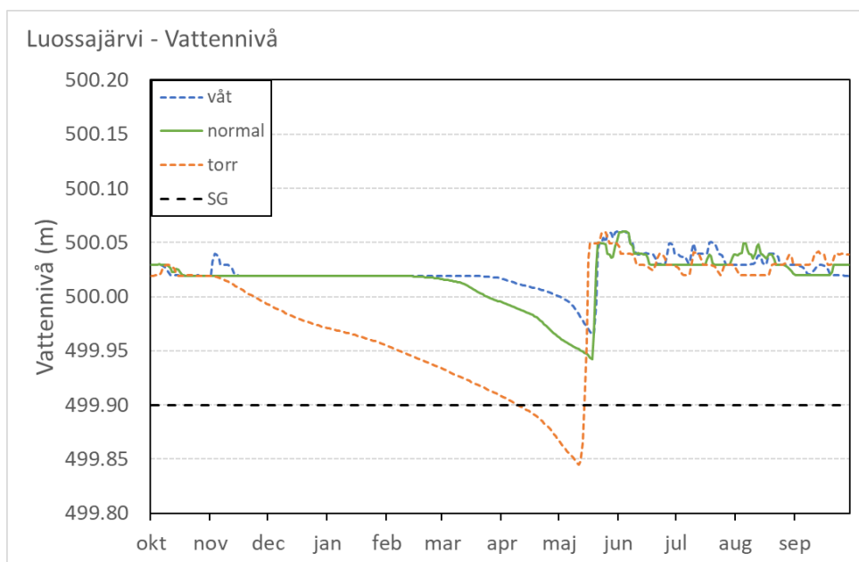
Figur 9-1. Vattennivåscenarier för Luossajärvi för det tre typåren: torrår (orange), normalår (grön) och våtår (blå) samt sänkingsgränsen (SG) som vattennivån få inte underskrider. Under perioder med liten variation i vattennivån fluktuerar nivån på cm-skala vilket ses som ett brus i kurvorna.
