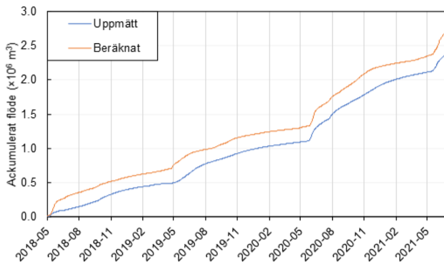
Figur 8-3. Uppmätta och beräknade flöden vid AVA15. (a) Hydrograf ( \text{m}^3/\text{s} ) (b) Ackumulerat flöde ( \times 10^6 \text{m}^3 ).
