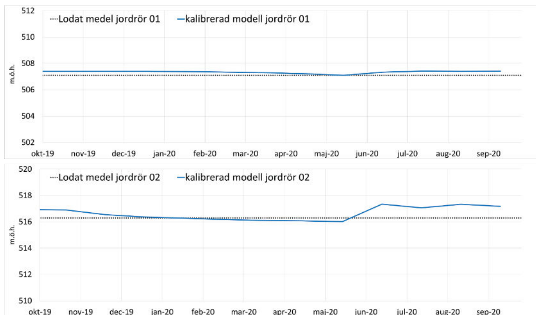
Figur 10-24. Modellerade och uppmätta grundvattennivåer för två av de jordrör som lodades vintern 2020/2021.
