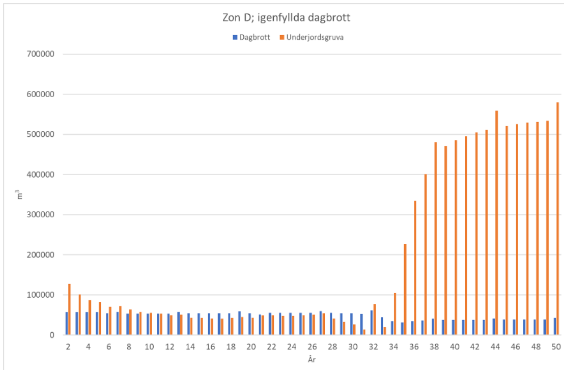
Figur 11-44. Inflödande vattenvolymer ( m^3/år ) till dagbrott och underjordsgruva i D-zonen för fallet med igenfyllda dagbrott. Om nettoflödet är positivt sker en inströmning av vatten, om det är negativt sker en utströmning av vatten.
