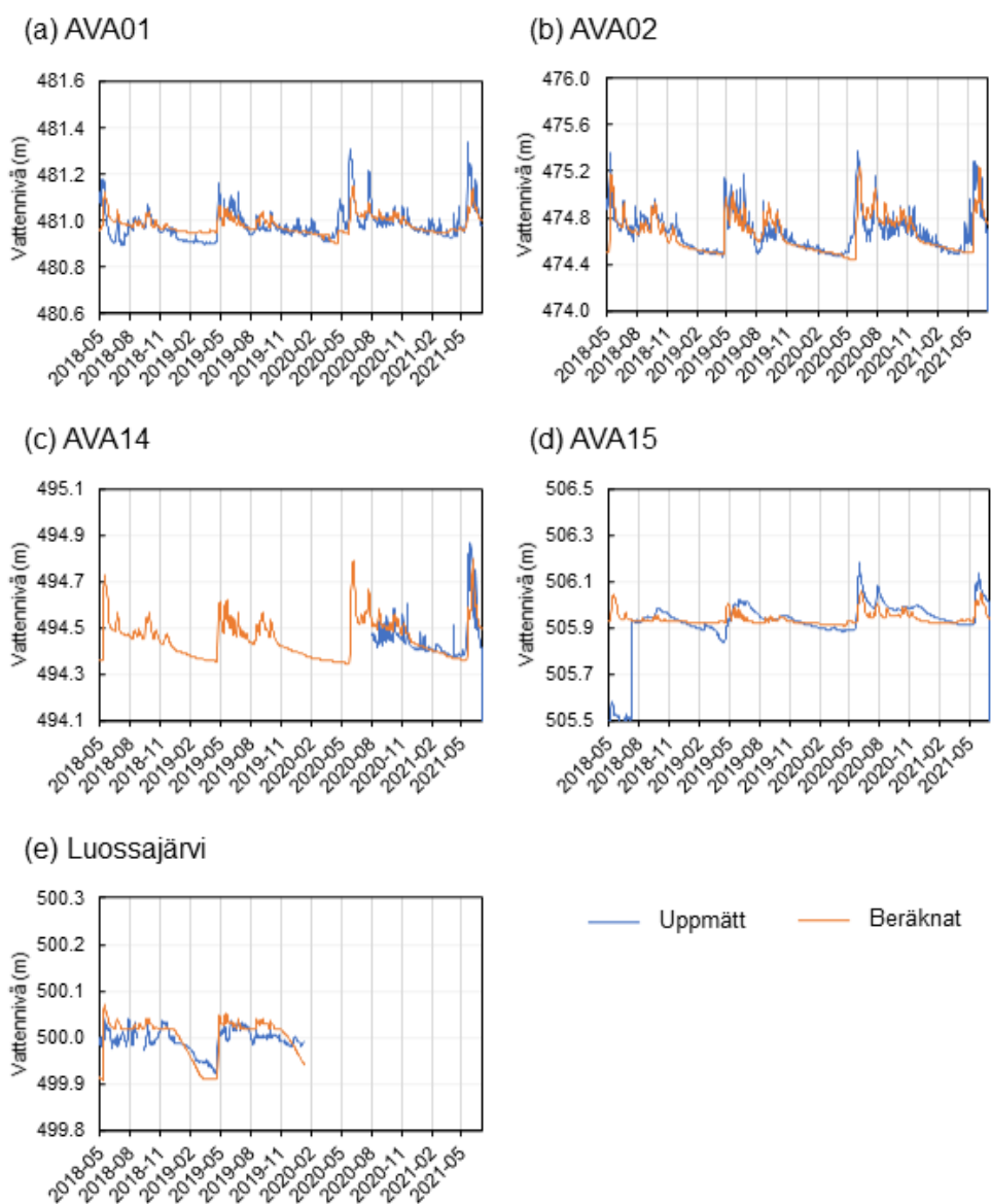
Figur 8-5. Grafer som visar de uppmätta och beräknade vattennivåerna (m) vid observationspunkterna: (a) AVA01, (b) AVA02, (c) AVA14, (d) AVA15 samt i (e) Luossajärvi.
