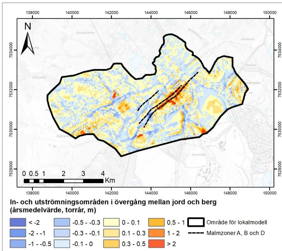
Figur 11-14. Beräknade in- och utströmningsområden vid övergången mellan jord och berg för dagens förhållanden under ett torrår. Resultat redovisas som årsmedelvärde.
