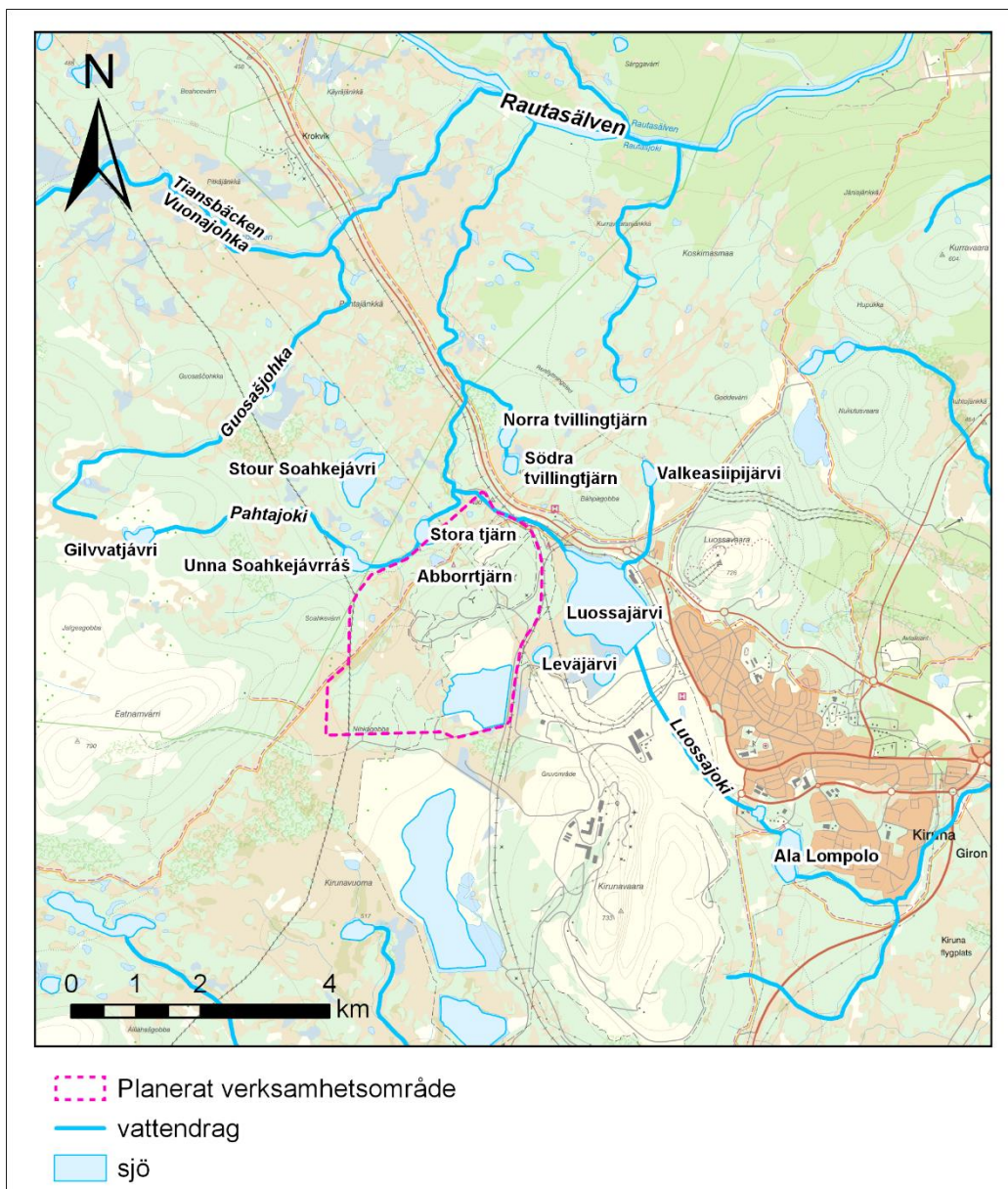
Figur 4-2. Ytvattenförekomster i Kiruna och Viscaria-området.
