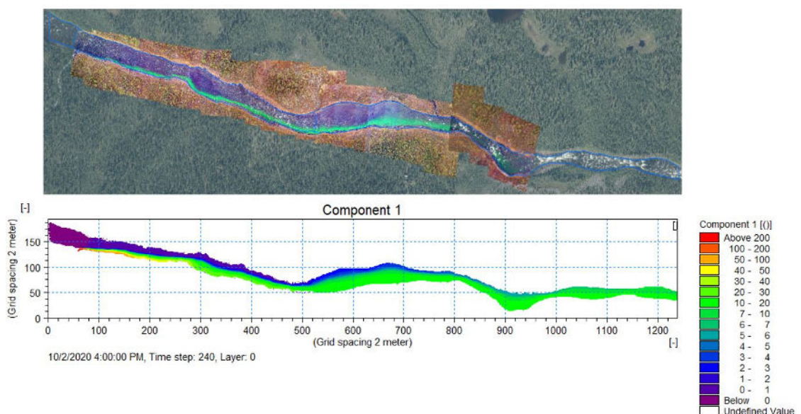
Figur 8-15. Simulerad spridning av ett konservativt ämne (nedre bilden) jämfört med spårämnesförsöket (övre bilden).
