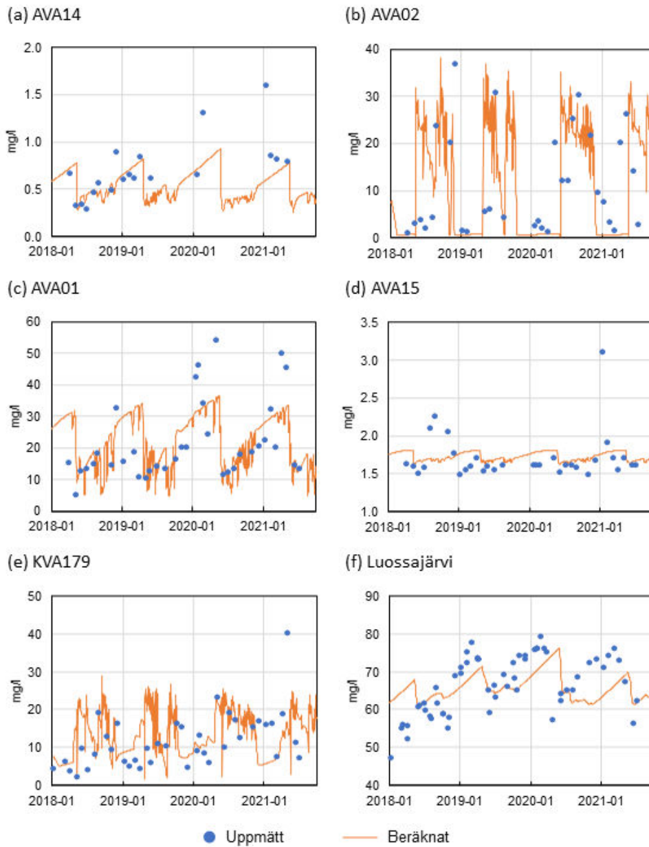
Figur 8-8. Uppmätta och beräknade klorid (Cl) halter (mg/l): (a) AVA14, (b) AVA02, (c) AVA01, (d) AVA15, (e) KVA179 och (f) Luossajärvi.
