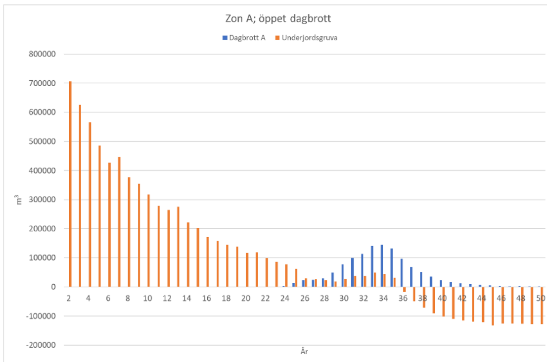
Figur 11-39. Inflödande vattenvolymer (m 3 /år) till dagbrott och underjordsgruva i A-zonen för fallet med öppna dagbrott. Om nettoflödet är positivt sker en inströmning av vatten, om det är negativt sker en utströmning av vatten.
