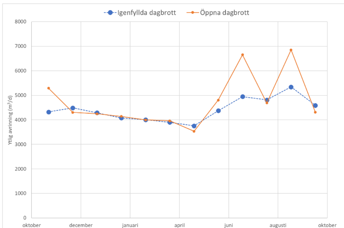
Figur 11-46. Total avrinning från område 2, 3, 6, 7a, 7b, 8, 9 och 12 för de två fallen med öppna och igenfyllda dagbrott.
