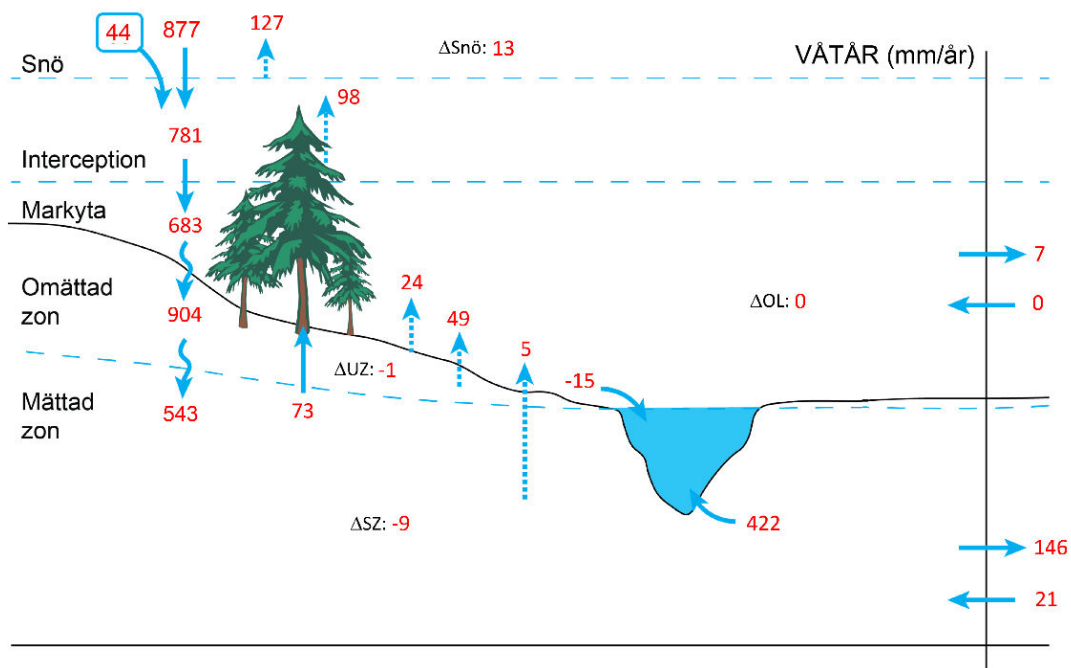
Figur 11-2. Vattenbalans i mm/år över modellerat våttår.
