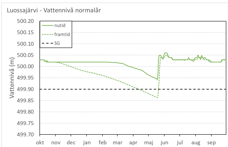
Figur 9-3. Jämförelse av förändringen av vattennivån i Luossajärvi för nutids- (heldragen grön linje) och framtidsscenarioer (streckad grön linje) för ett normalår i förhållande till sänkingsgränsen (SG – streckad svart linje).
