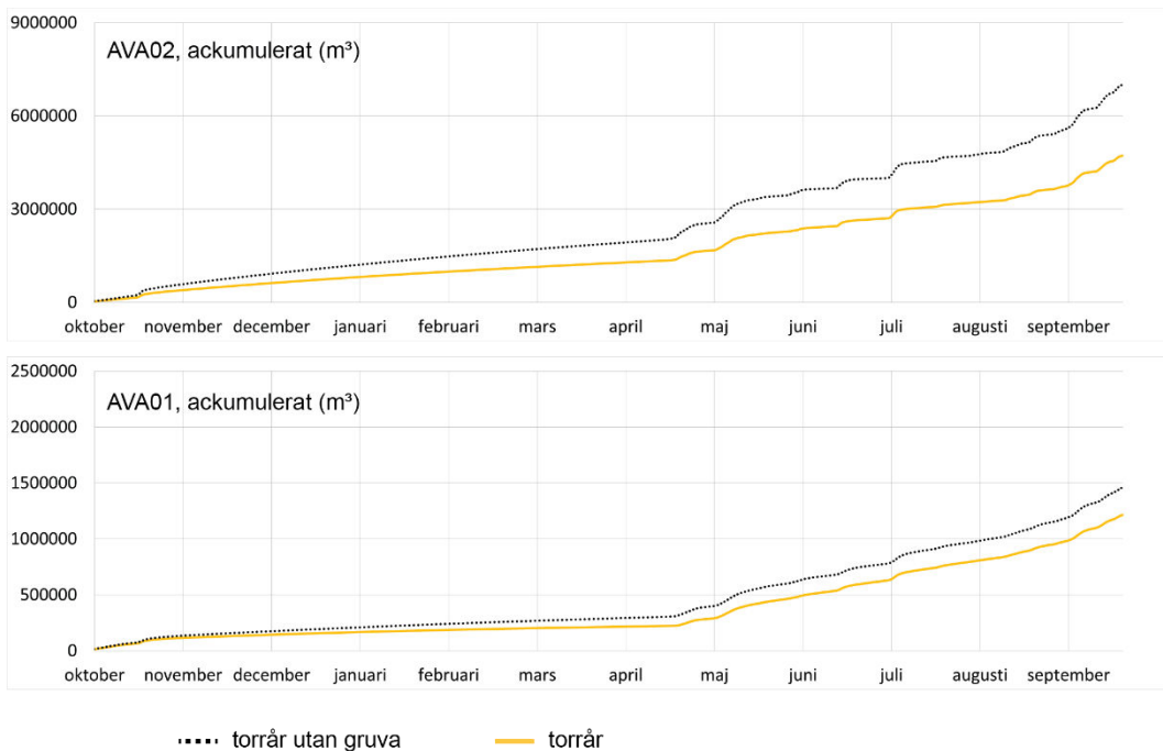
Figur 11-32. Ackumulerad avrinning för ett torrår i AVA02 i Pahtajokisystemet samt AVA01 i Tvillingsjösystemet vid framtida gruvdrift, samt för det opåverkade referensfallet vid torrår.
