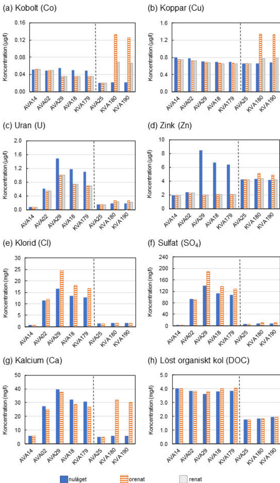
Figur 9-8. Modellerade normalårshalter där brädning sker i Rautas (R i Figur 9-6) för scenarierna nuläget, orenat och renat: (a) Co, (b) Cu, (c) U, (d) Zn, (e) Cl, (f) SO 4 , (g) Ca och (h) DOC. Figuren inkluderar vattendragen vid Pahtajoki, vänster om streckad linje och Rautasälven, höger om streckad linje.
