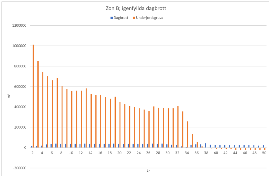
Figur 11-42. Inflödande vattenvolymer ( m^3/\text{år} ) till dagbrott och underjordsgruva i B-zonen för fallet med igenfyllda dagbrott. Om nettoflödet är positivt sker en inströmning av vatten, om det är negativt sker en utströmning av vatten.
