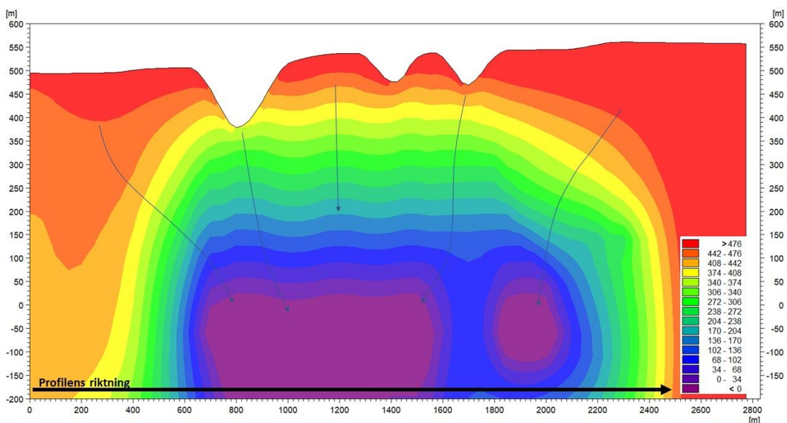
Figur 11-29. Beräknad grundvattennivå på olika djup i berget utmed profil A vid framtida gruvdrift.
