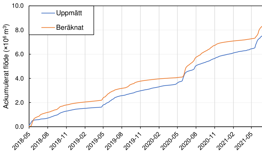
Figur 8-1. Uppmätta och beräknade flöden vid AVA01. (a) Hydrograf ( \text{m}^3/\text{s} ) (b) Ackumulerat flöde ( \times 10^6 \text{m}^3 ).
