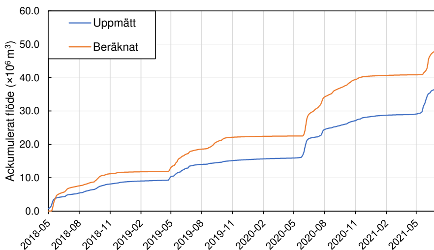
Figur 8-2. Uppmätta och beräknade flöden vid AVA02. (a) Hydrograf ( \text{m}^3/\text{s} ) (b) Ackumulerat flöde ( \times 10^6 \text{m}^3 ).
