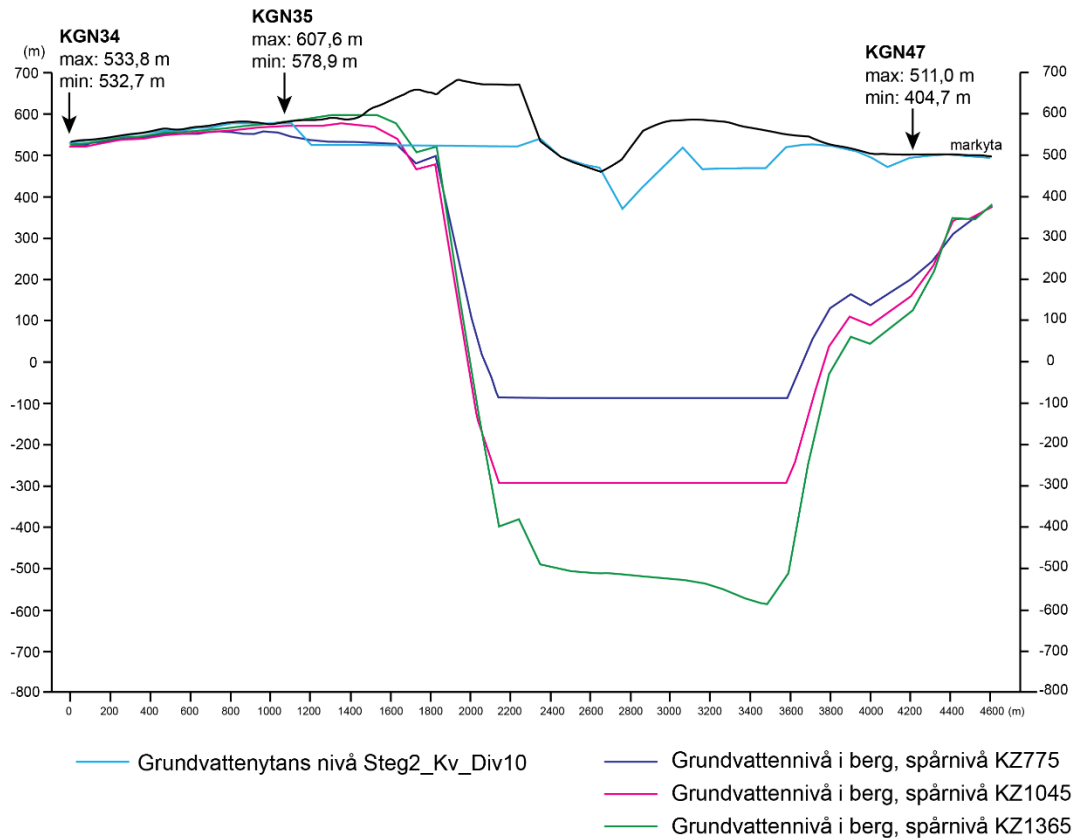
Figur 10-5. Beräknad grundvattenyta och grundvattennivå på olika djup i berget för profil 1, KGN34-KGN47, från beräkningar i steg 2, fall Steg2_Kv_Div10. Om grundvattennivån i beräkningslaget hamnar under beräkningslagrets nedre nivå visas grundvattennivån som ett rakt streck, detta inträffar ca 2000 m in i profilen för de två lager som innehåller de två övre spårnivåerna.
