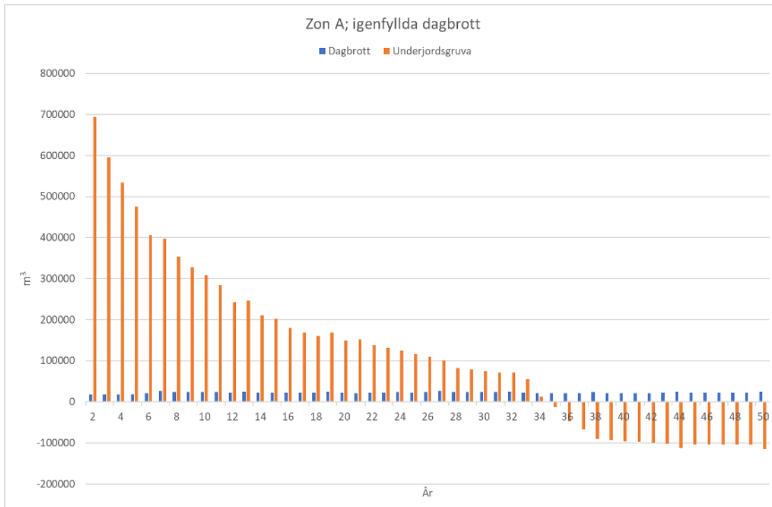
Figur 11-40. Inflödande vattenvolymer (m 3 /år) till dagbrott och underjordsgruva i A-zonen för fallet med igenfyllda dagbrott. Om nettoflödet är positivt sker en inströmning av vatten, om det är negativt sker en utströmning av vatten.
