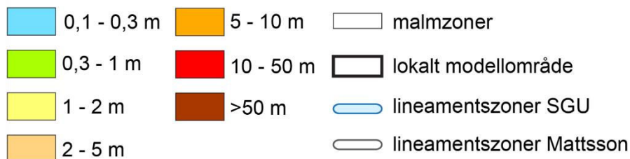
Figur 11-26 Påverkan på grundvattenytan för normalåret med en gräns för avsänkning på 10 cm.
