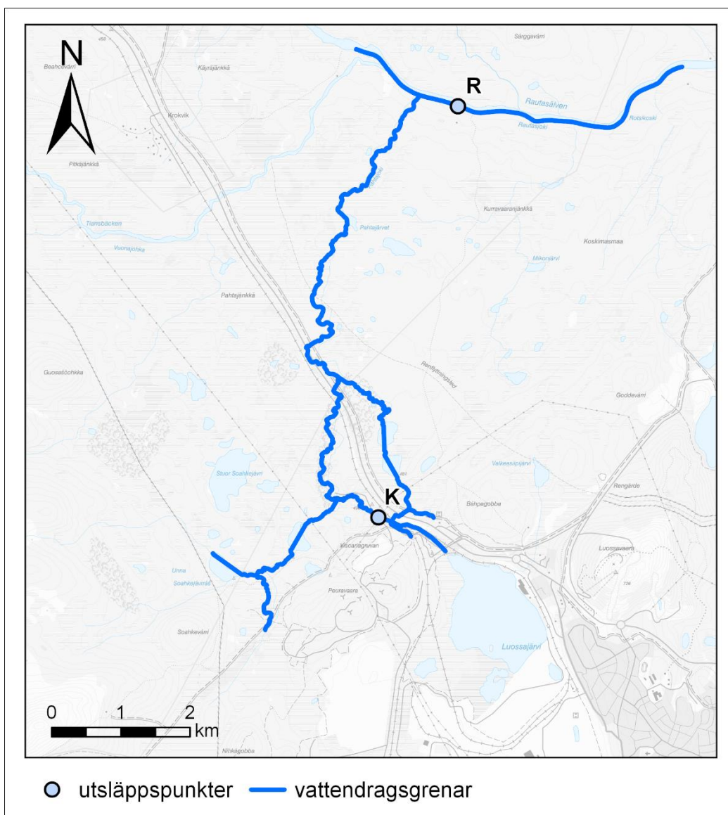
Figur 9-6. Placering av bräddningspunkterna för framtidsscenerierna där bräddning sker i kanalen (K) eller i Rautas älv (R). AVA02 är den mätpunkt som ligger närmast bräddningspunkten K och KVA180 är den mätpunkt som ligger närmast bräddningspunkten R.
