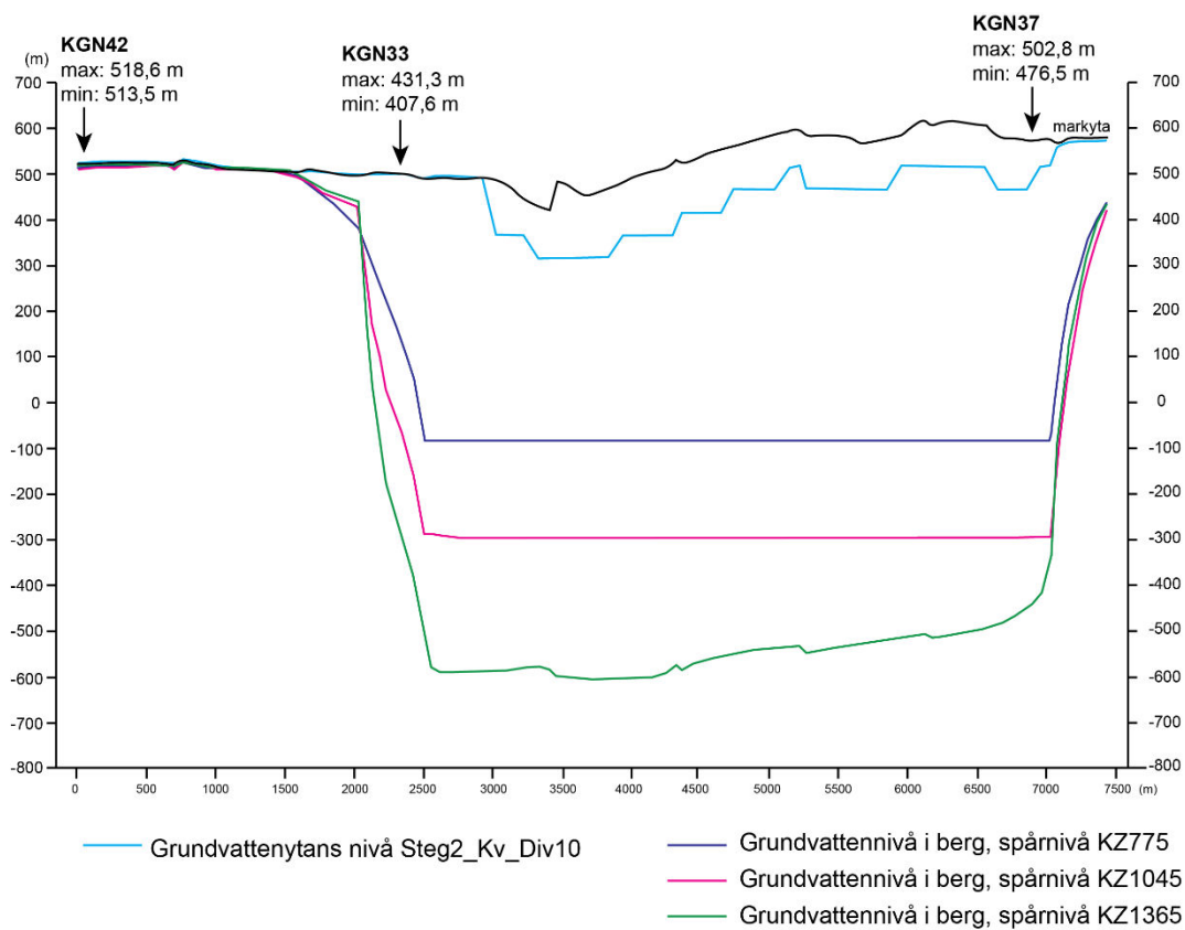
Figur 10-6. Beräknad grundvattenyta och grundvattennivåer på olika djup i berget för profil 2, KGN42-KGN37, från beräkningar i steg 2, fall Steg2_Kv_Div10. Om grundvattennivån i beräkningslagret hamnar under beräkningslagrets nedre nivå visas grundvattennivån som ett rakt streck, detta inträffar ca 2500 m in i profilen för de två lager som innehåller de två övre spårnivåerna.
