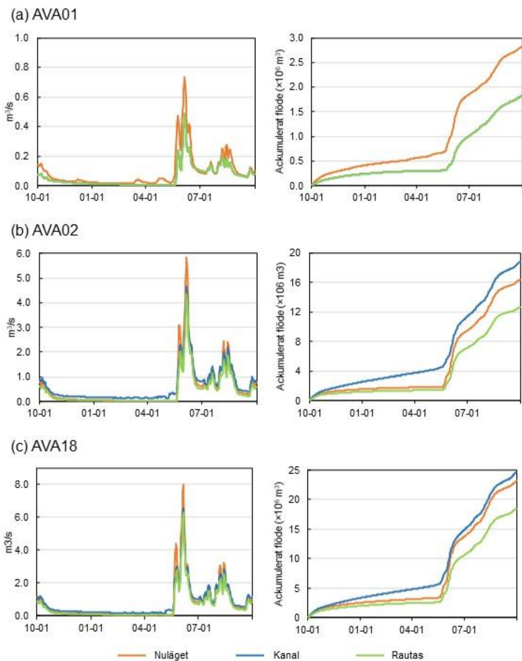
Figur 9-5. Beräknade flöden för Nuläget (orange linje), och de två framtidsscenerierna Kanal (blå linje) och Rautas (grön linje) för mätpunkterna AVA01, AVA02 och AVA18. Graferna till vänster i figuren visar flöde ( \text{m}^3/\text{s} ) över ett hydrologiskt år medan graferna till höger visar ackumulerat flöde över ett hydrologiskt år. För mätpunkt AVA01 sammanfaller flödena för framtidsscenerierna, dvs de är identiska. Figur 9-6 visar placering av bräddpunkterna för Kanal-scenariot och Rautas-scenariot.
