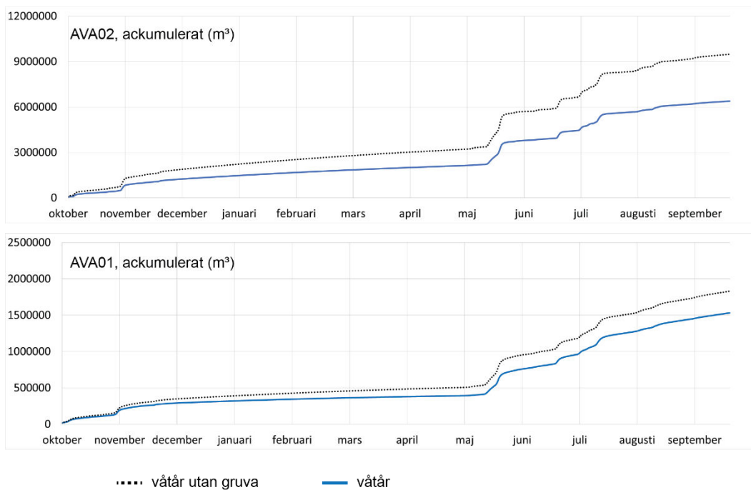
Figur 11-33. Ackumulerad avrinning för ett våtår i AVA02 i Pahtajokisystemet samt AVA01 i Tvillingsjösystemet vid framtida gruvdrift, samt för det opåverkade referensfallet vid våtår.
