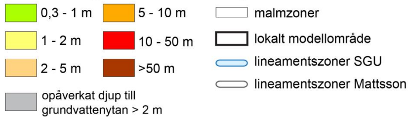
Figur 11-21. Påverkansområde vid tömning av befintlig gruva och vid fullt utbruten gruva i Fas 3, normalår. Påverkade områden med större djup till grundvattenytan än 2 m under opåverkade förhållanden är gråmarkerade.
