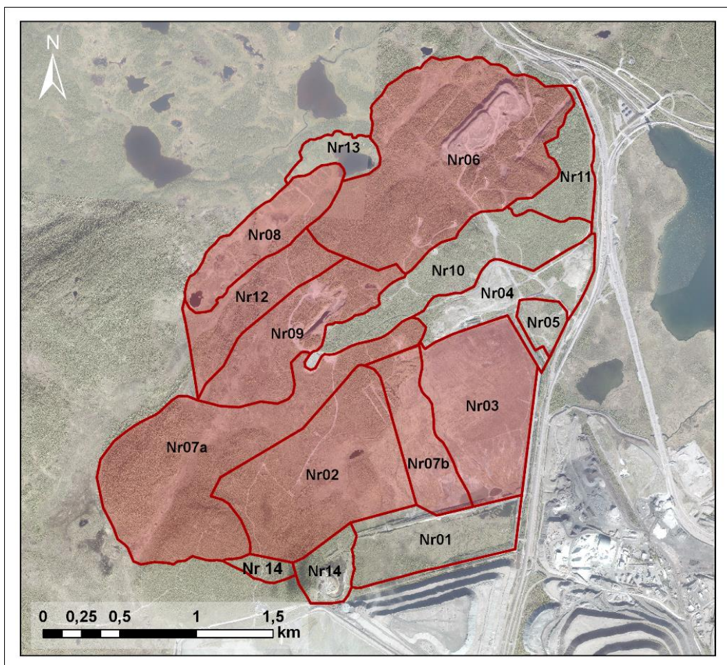
Figur 11-45. Totala avrinning har beräknats för det gemensamma området som utgörs av delavrinningsområde 2, 3, 6, 7a, 7b, 8, 9 och 12.
