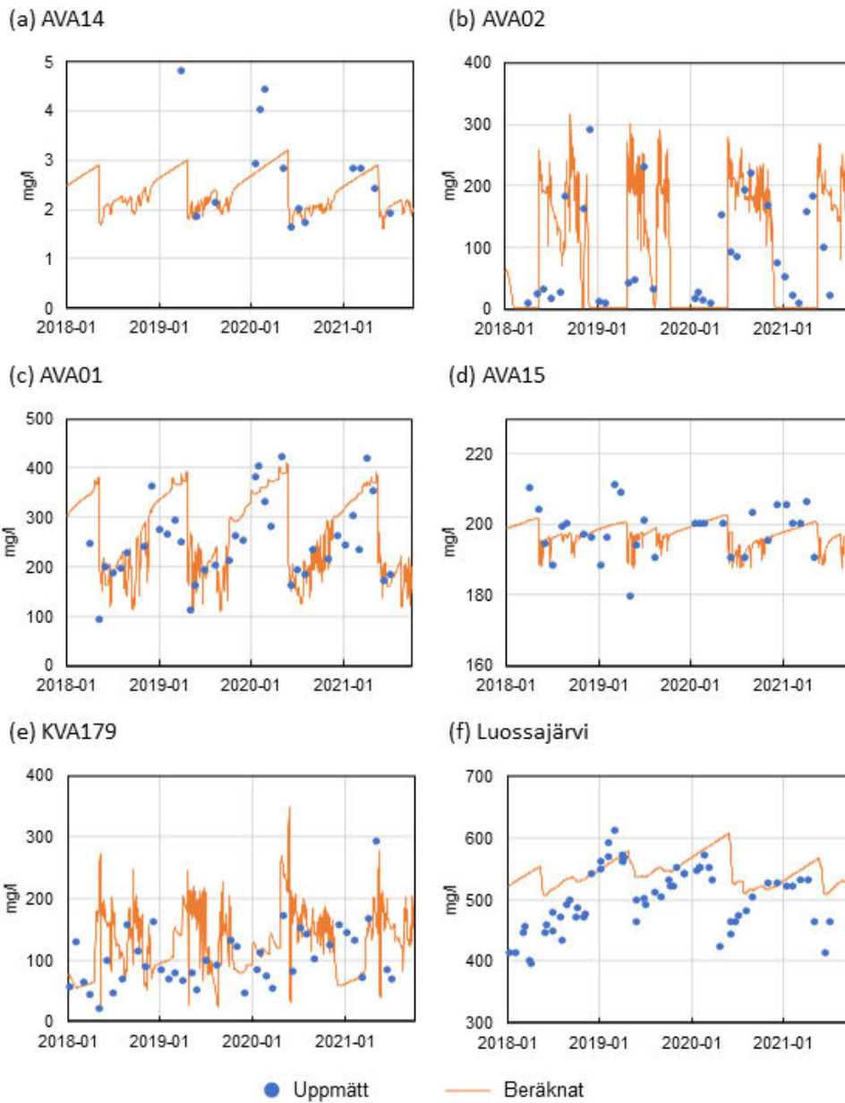
Figur 8-11. Uppmätta och beräknade halter av sulfat ( \text{SO}_4 ) (mg/l): (a) AVA14, (b) AVA02, (c) AVA01, (d) AVA15, (e) KVA179 och (f) Luossajärvi.
