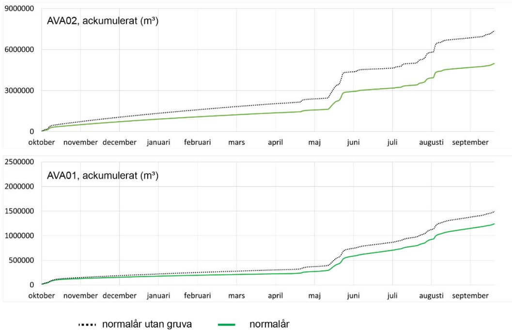
Figur 11-31. Ackumulerad avrinning för ett normalår i AVA02 i Pahtajokisystemet samt AVA01 i Tvillingsjösystemet vid framtida gruvdrift, samt för det opåverkade referensfallet vid normalår.
