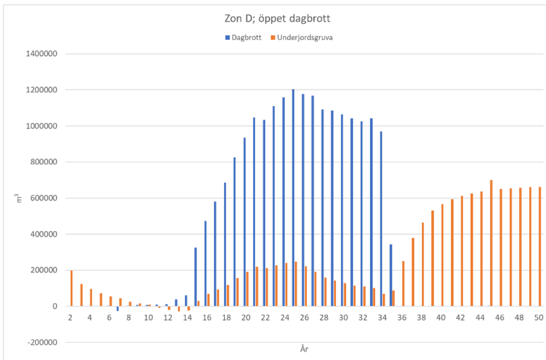
Figur 11-43. Inflödande vattenvolymer ( m^3/år ) till dagbrott och underjordsgruva i D-zonen för fallet med öppna dagbrott. Om nettoflödet är positivt sker en inströmning av vatten, om det är negativt sker en utströmning av vatten.
