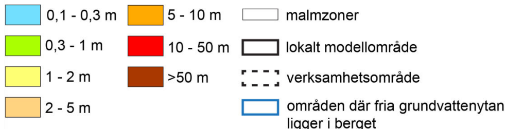
Figur 11-27. Påverkan på grundvattenytan för normalåret med en gräns för avsänkning på 10 cm. De områden inom påverkansområdet där grundvattenytan hamnar i berget har ringats in med svarta linjer. I de områden inom påverkansområdet som inte är markerade ligger grundvattenytan i jordlagren.
