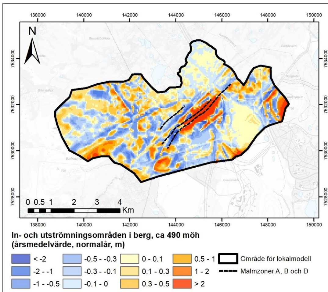
Figur 11-16. Beräknade in- och utströmningsområden i berg på nivån ca 490 m ö.h. för dagens förhållande under ett normalår. Resultat visas för årsmedelvärdet.
