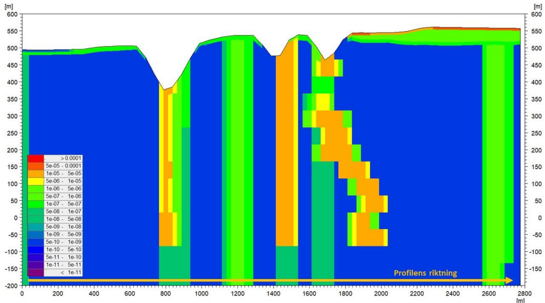
Figur 11-28. Vertikal hydraulisk konduktivitet för en utbyggd gruva, längs med profil A enligt Figur 11-6.
