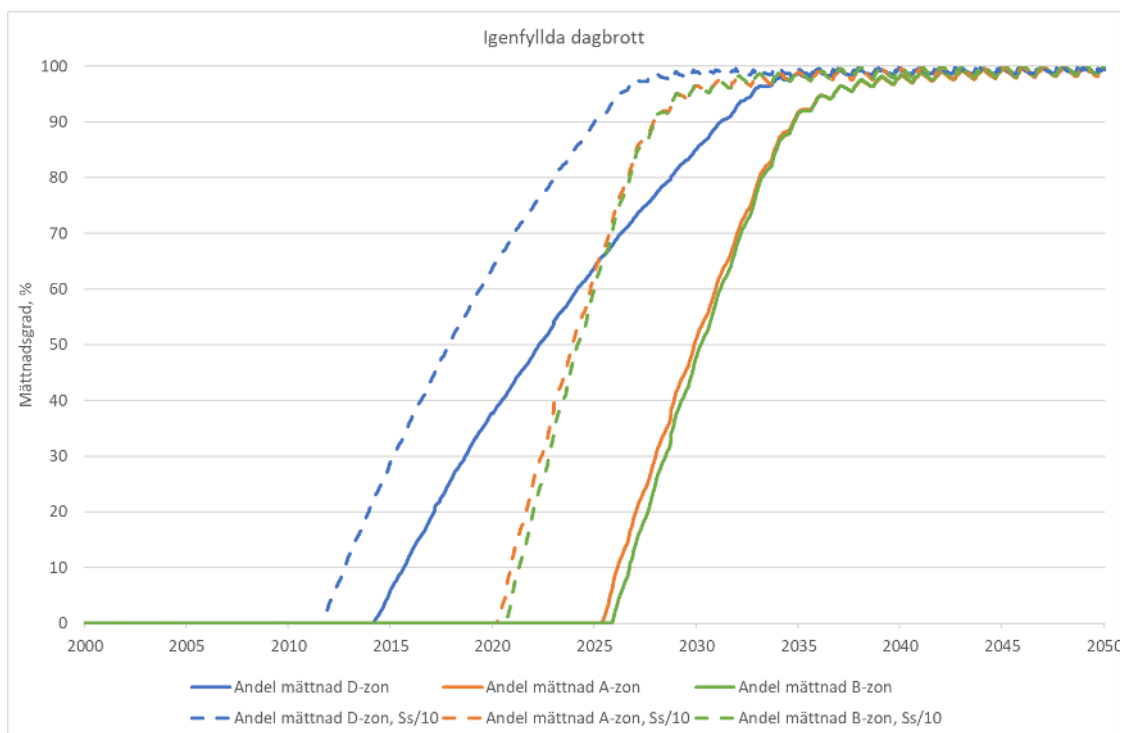
Figur 11-38. Återmättnadsförlopp i fallet med igenfyllda dagbrott. Figuren visar andelen av dagbrotten som är vattenfyllda i förhållande till tröskelnivån, dvs den nivå där ytvatten börjar flöda ut ur dagbrottssjöarna.
