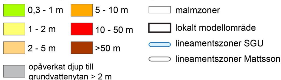
Figur 11-25. Påverkansområde vid tömning av befintlig gruva och vid fullt utbruten gruva i Fas 3, våtår. Påverkade områden med större djup till grundvattenytan än 2 m under opåverkade förhållanden är gråmarkerade.
