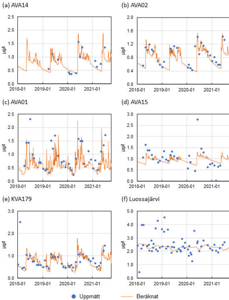
Figur 8-7. Uppmätta och beräknade koppar (Cu) halter ( \mu\text{g/l} ): (a) AVA14, (b) AVA02, (c) AVA01, (d) AVA15, (e) KVA179 och (f) Luossajärvi.
