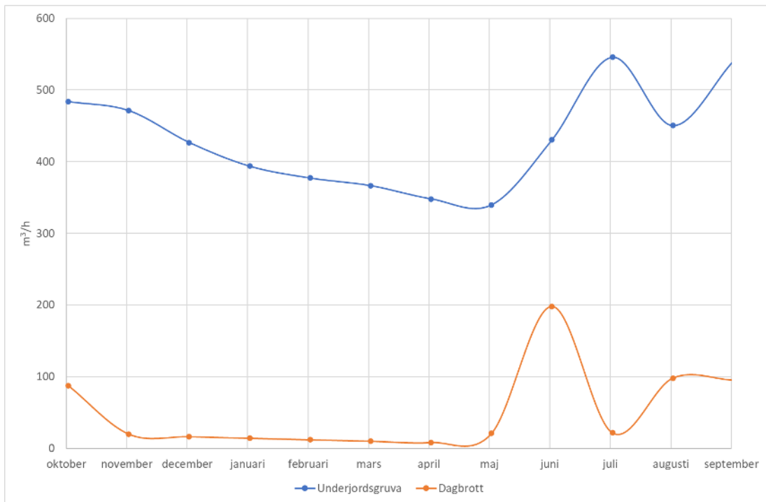
Figur 11-34. Inläckage till underjordsgruva respektive dagbrott för en årscykel, normalår.
