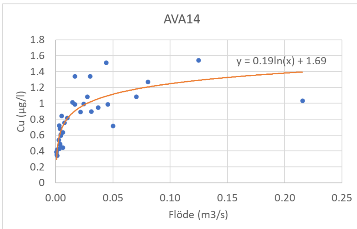
Figur 7-1. Uppmätt Cu-halt och uppmätt flöden vid AVA14.
