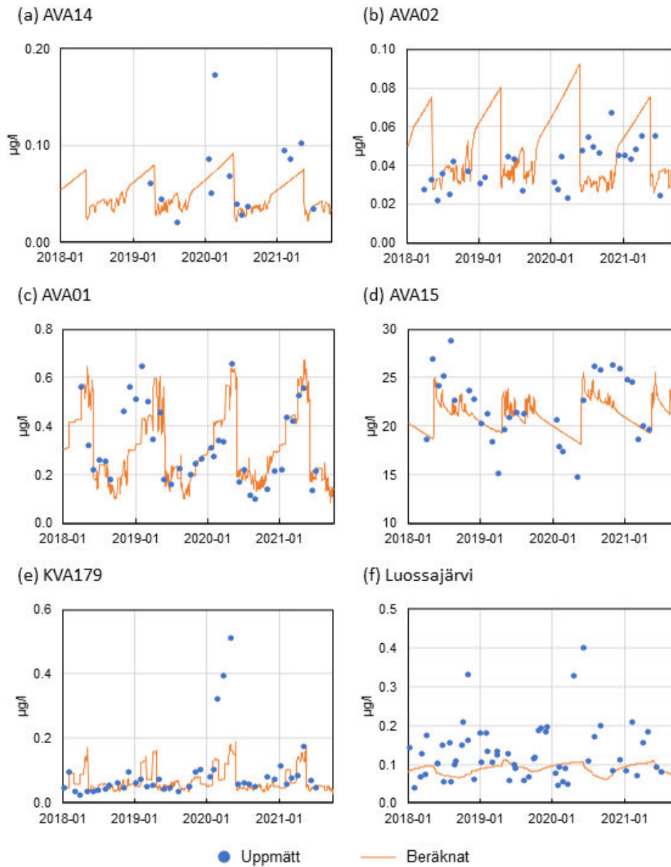
Figur 8-6. Uppmätta och beräknade kobolt (Co) halter ( \mu\text{g/l} ): (a) AVA14, (b) AVA02, (c) AVA01, (d) AVA15, (e) KVA179 och (f) Luossajärvi.
