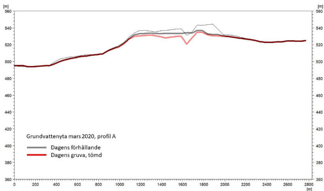
Figur 11-8. Grundvattenytans läge i mars 2020 längs profil A enligt Figur 11-6. Den mörkgråa linjen visar grundvattenytans läge för dagens förhållande, och den röda visar motsvarade för fallet med dagens gruva tömd på vatten.
