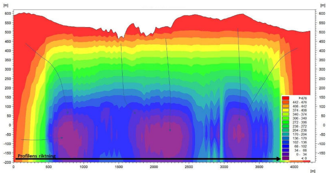
Figur 11-30. Beräknad grundvattennivå på olika djup i berget utmed profil B för de tre olika gruvscenarierna.
