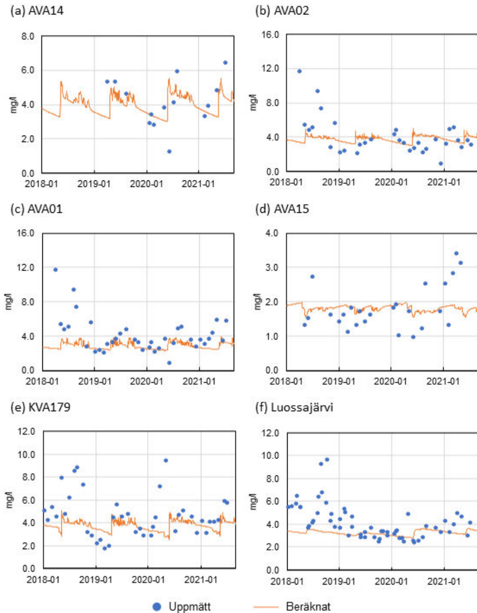
Figur 8-13. Uppmätta och beräknade halter av löst organiskt kol (DOC) (mg/l): (a) AVA14, (b) AVA02, (c) AVA01, (d) AVA15, (e) KVA179 och (f) Luossajärvi.
