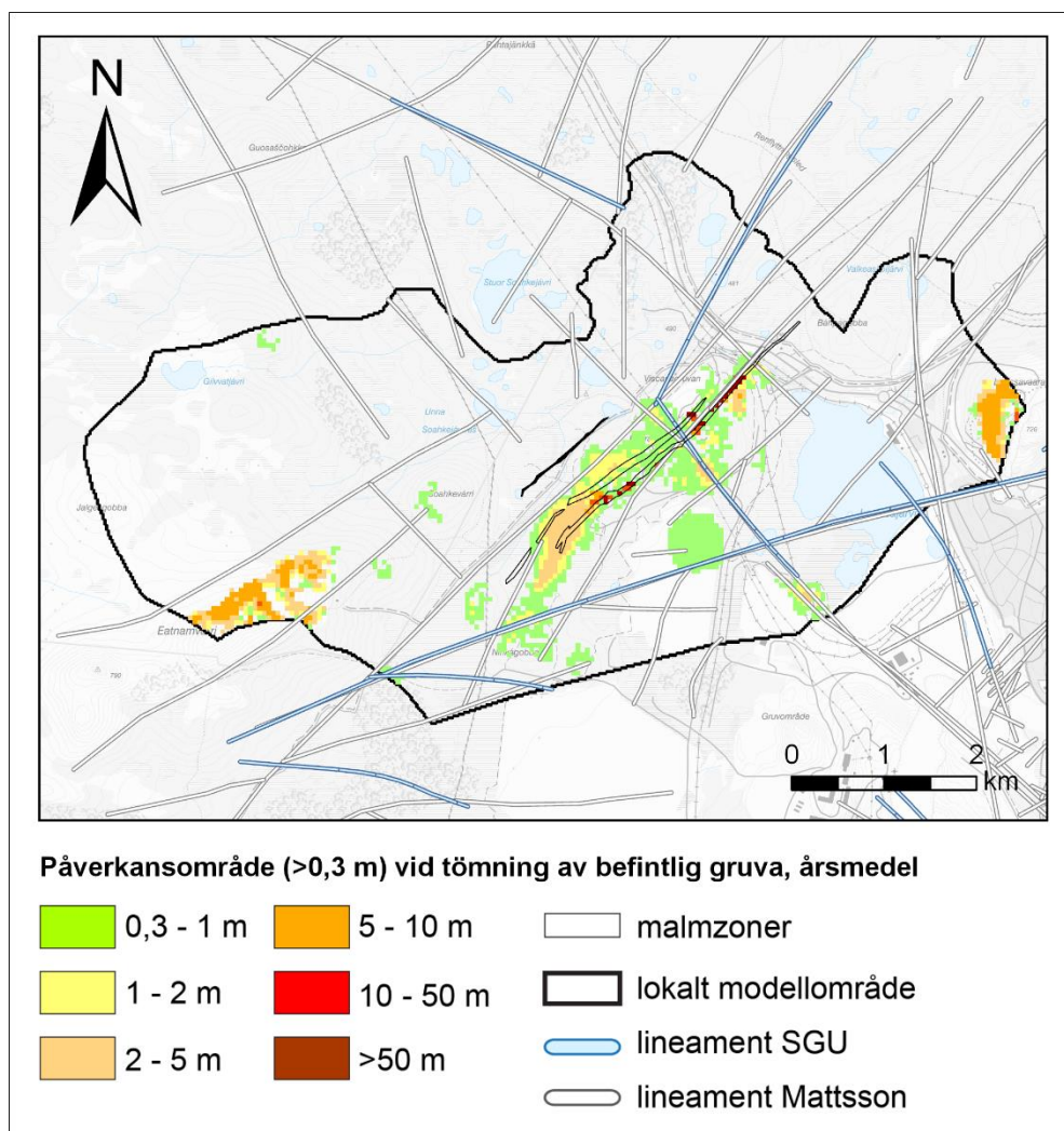
Figur 10-23. Beräknat årsmedel på avsänkning av grundvattenytan när gruvan i AB-zonen torrläggs. Områden som sänks av mer än 30 cm är markerade i kartan.
