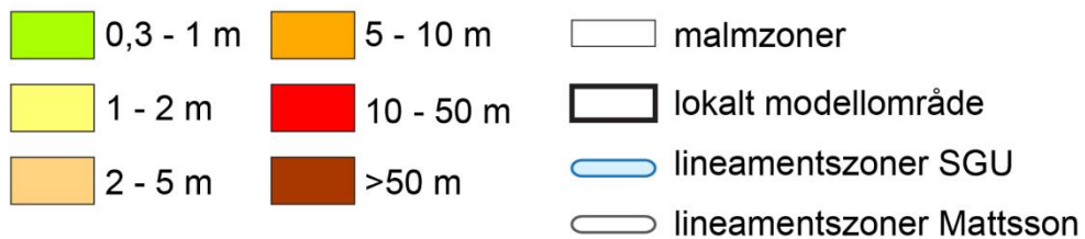
Figur 11-24. Påverkansområde vid tömning av befintlig gruva och vid fullt utbruten gruva i Fas 3, våtår.
