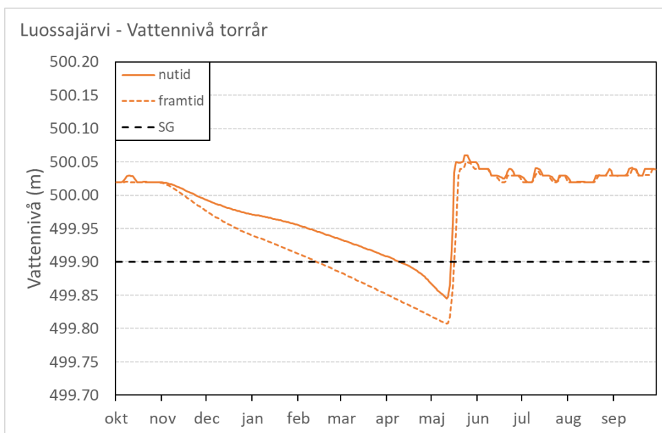
Figur 9-2. Jämförelse av förändringen av vattennivån i Luossajärvi för nutids- (heldragen orange linje) och framtidsscenarioer (streckad orange linje) för ett torrår i förhållande till sänkingsgränsen (SG – streckad svart linje).
