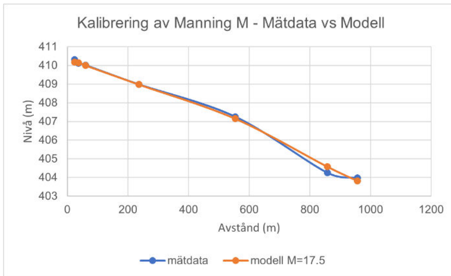
Figur 8-14. Uppmätta och modellerade vattennivåer i Rautasälven.
