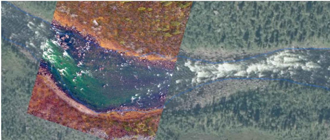
Figur 8-16. Drönarbild av höljan 1800 m nedströms Pahtajokiutloppet. Enligt simuleringarna uppnås full omblandning strax nedströms höljan, dvs i den trånga fallsträckan.
